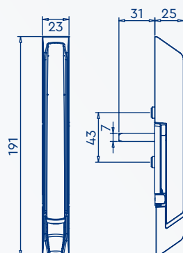
MAC392 · DESENHO TÉCNICO · COTAS EM mm
