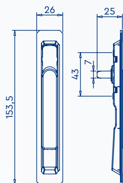
MAC393 · DESENHO TÉCNICO · COTAS EM mm
