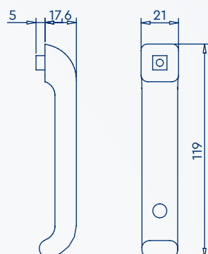
FEC670 · DESENHO TÉCNICO · COTAS EM mm
