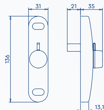
FEC675 · DESENHO TÉCNICO · COTAS EM mm
